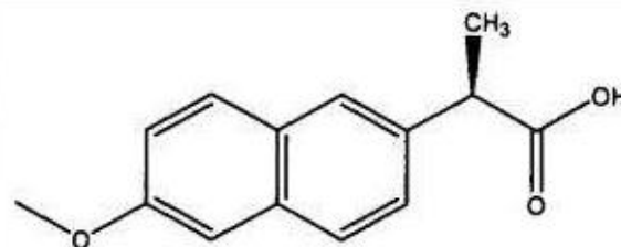
(R)-Naproxen
