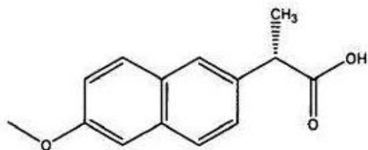
S-Naproxen
